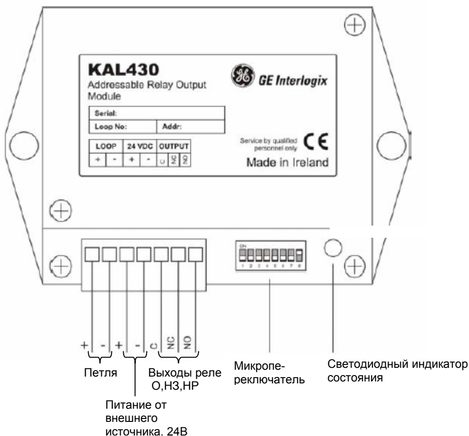
Рисунок 1. Подключение модуля KAL430.
