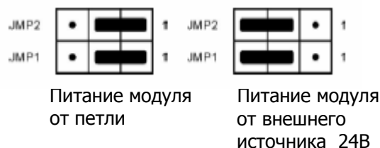
Рисунок 2. Выбор способа питания модуля.
